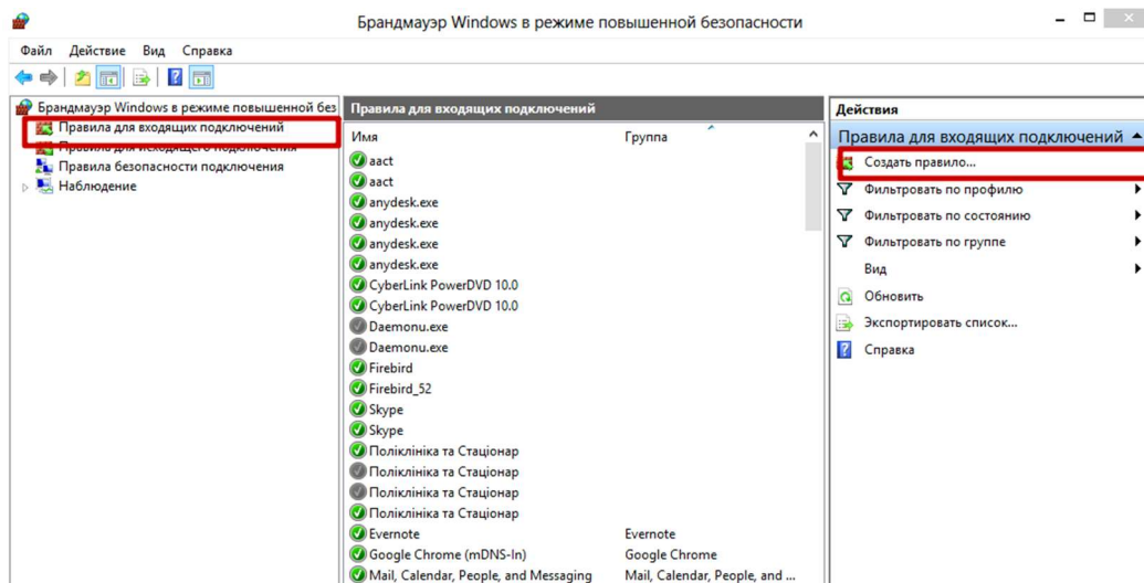
Рисунок 8 – «Брандмауэр Windows».
