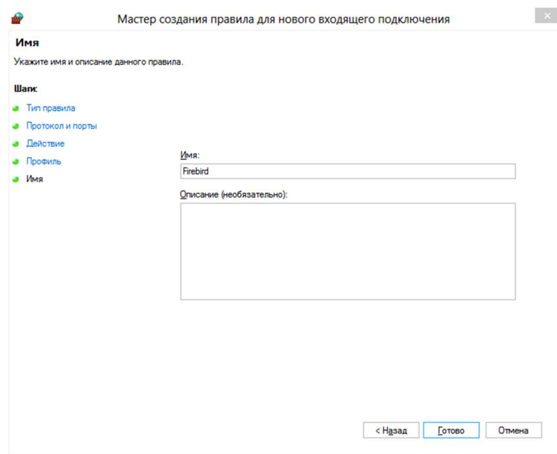
Рисунок 11 – Додавання порта
