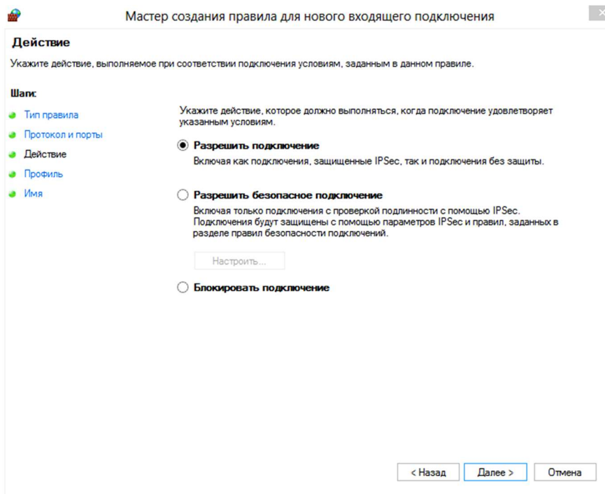
Рисунок 10 – Додавання порта
