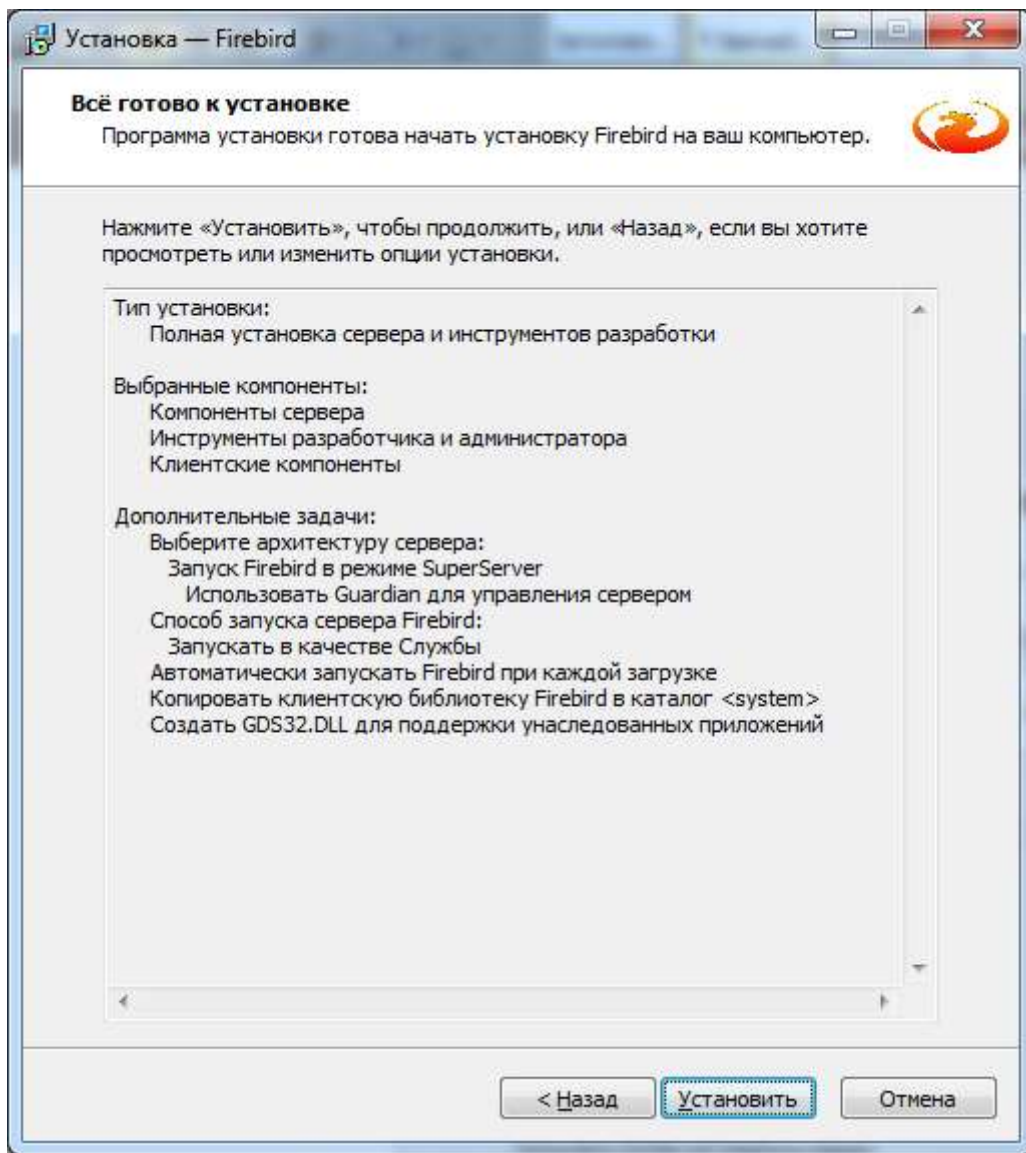
Рис. 1.7 – Вікно з інформацією про дії інстальатора
