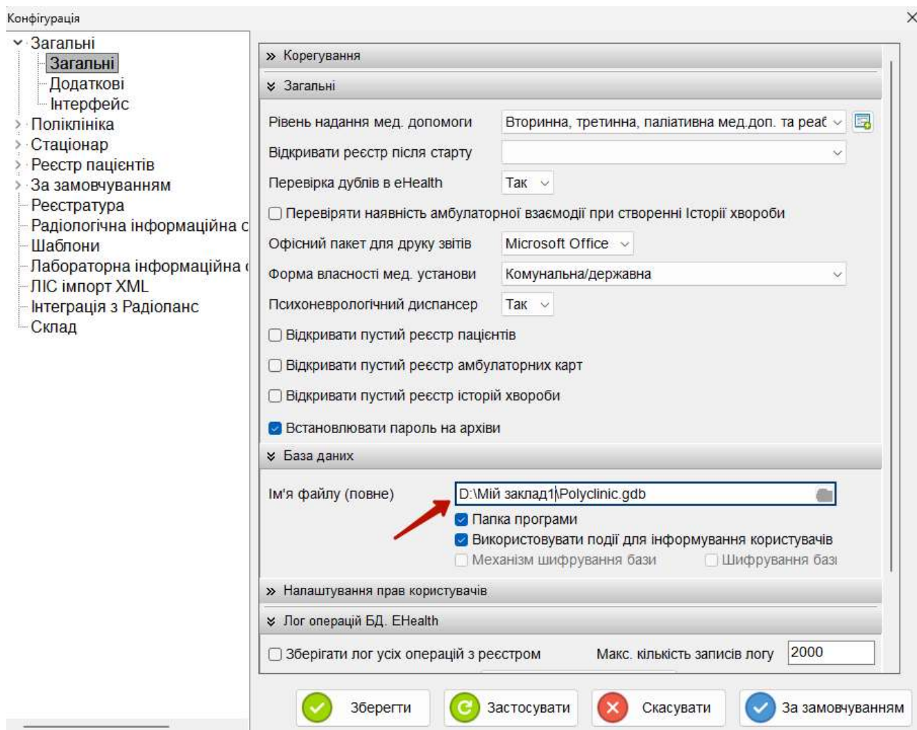
Рисунок 3.3 – Режим конфігурації
