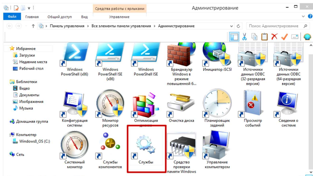
Рисунок 6 – Апплет “Администрирование”.
